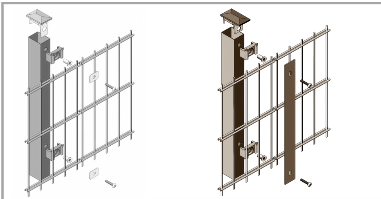
mit Klemmplättchen (Typ PFK)
